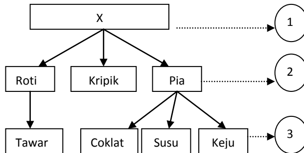
Gambar 1 Alur Logika Secara Sederhana Metode Back Tracking
