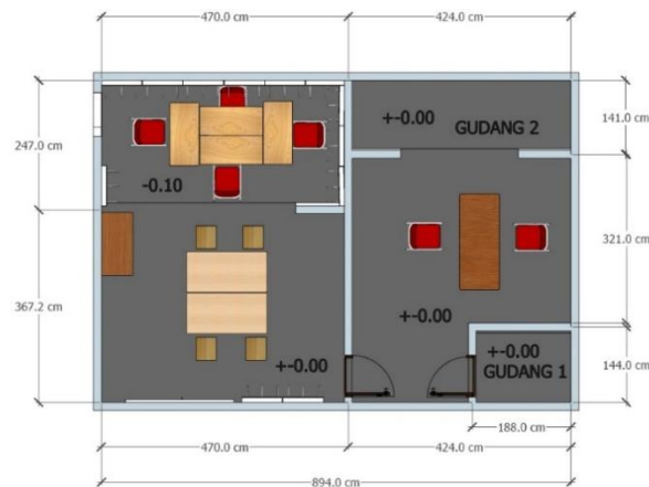
Gambar 4 : Layout Awal (Sumber : Brian, 2022)
