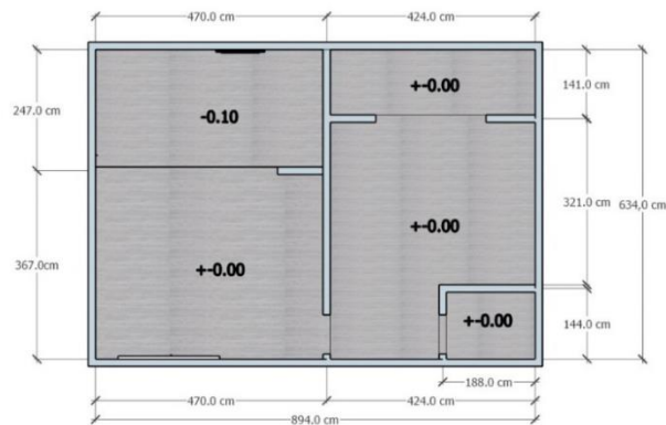
Gambar 3 : Floor Plan (Sumber : Brian, 2022)
