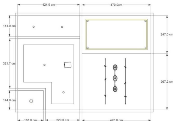
Gambar 18: Rencana Ceiling
