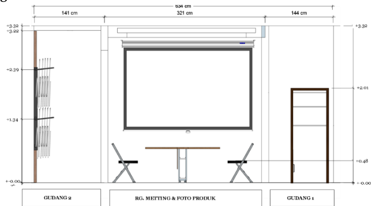
Gambar 9 : Potongan A-A2 (Sumber : Brian, 2022)
