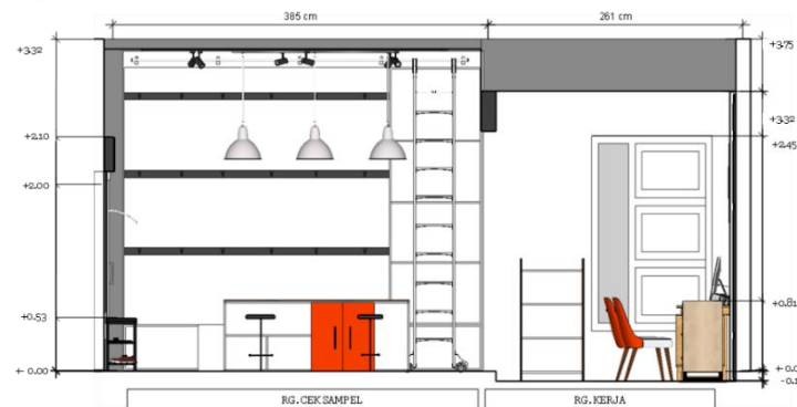
Gambar 8 : Gambar Potongan A-A1 (Sumber : Brian, 2022)
