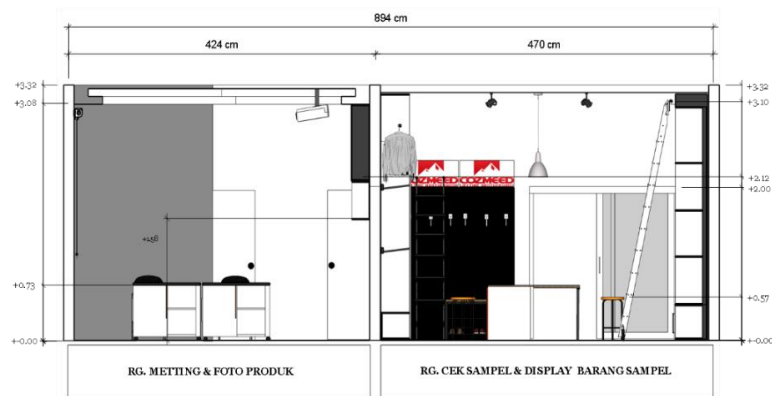
Gambar 11 : Potongan B-B2 (Sumber : Brian, 2022)
