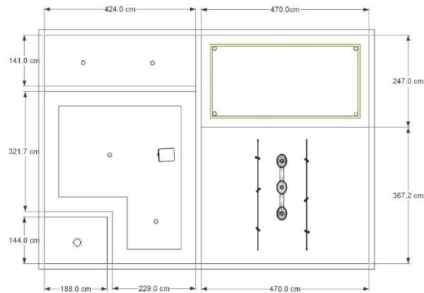
Gambar 6 : Ceiling Kantor (Sumber : Brian, 2022)
